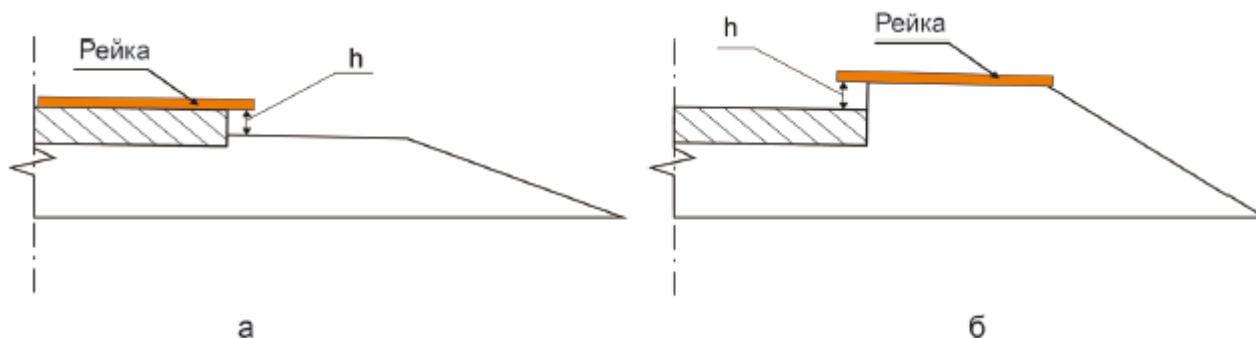
Рисунок 1 - Схема измерения величины занижения (возвышения) обочины и разделительной полосы:
